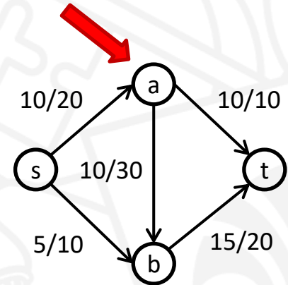
Fluxo Inviável
