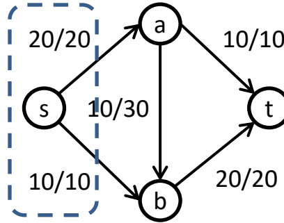
Fluxo Máximo
