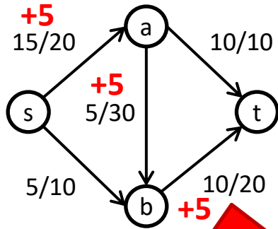
Fluxo Viável
